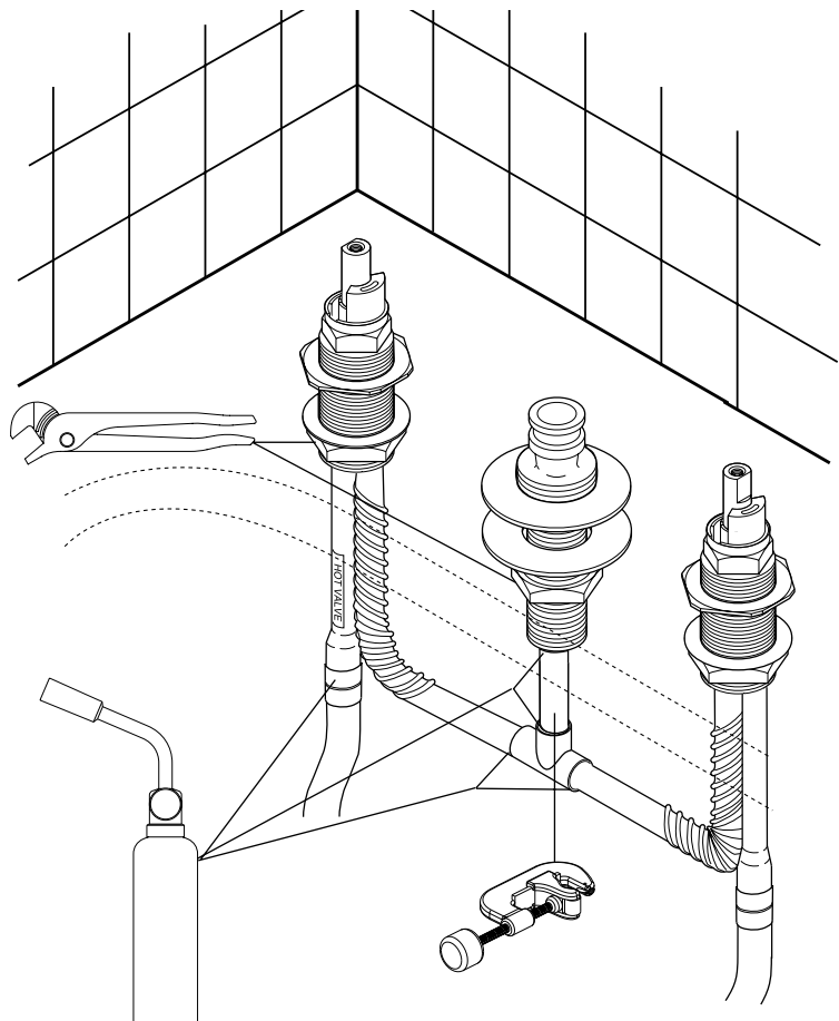
5/8" (15.9mm) O.D. Copper Tubing 5/8" (15.9 mm) D.E. Tubería de cobre Tube de cuivre de 5/8 po (15,9 mm) d.e.
