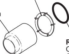
RP50879▲ Trim Sleeve Manga de franja Manchon de finition
