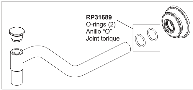
RP100325▲ Shower Arm & Flange Brazo de la regadera y brida Bras de douche et collerette
