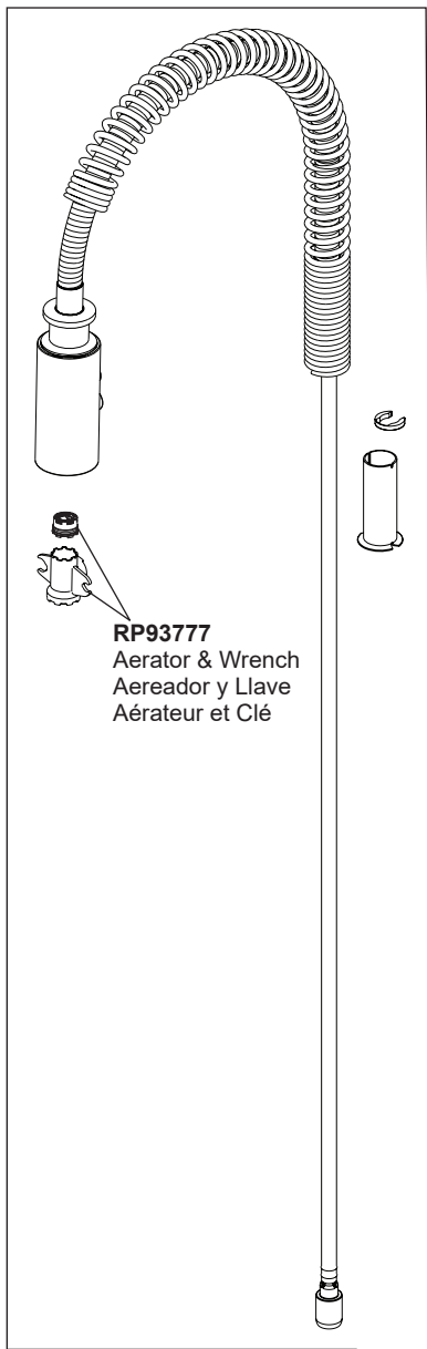
RP101728▲ Spring & Sprayer Assembly Ensemble de resorte y pulverizador Assemblage ressort et pulvérisateur
