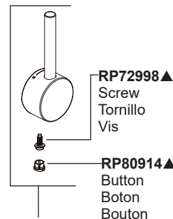
HLK177▲ Wood Handle Kit Mango con herraje Manette trousse
