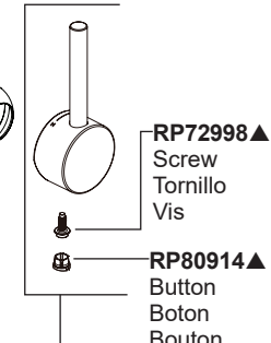
HLK175▲ Handle Kit Mango con herraje Manette trousse
