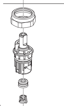
RP101069 Stem Unit Assembly, Seat & Spring, Bonnet Nut Ensemble de la Unidad del Vástago, Asiento y Resorte, Bonete Obturateur, siège et ressort, écrou à chapeau
