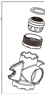
RP102039 Aerator & Wrench Aireador y Llave Aérateur et Clé
