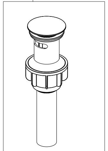
RP100137▲ Push Pop-UP with Overflow Control de rebose para desagües manuales Mécanique à poussoir avec trop-plein
