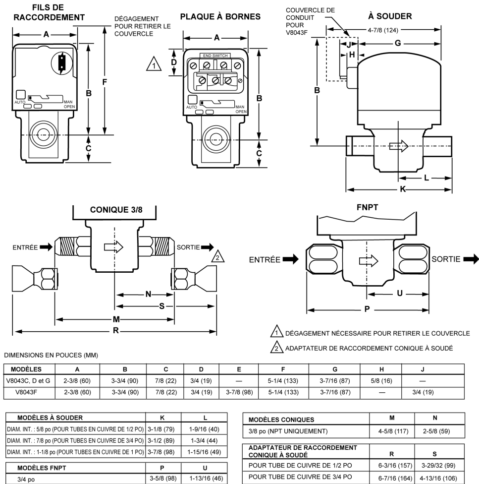
Fig 1. Dimensions en pouces (mm).
