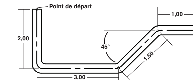
B – Tube courbé aux axes
